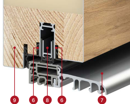
THERMO 78 ajtószárny keresztmetszete takaró tömítéssel és anélkül, alumínium küszöb
