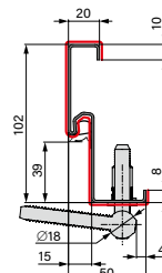
ACÉL SAROK AJTÓTOK
