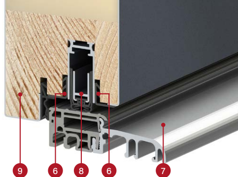
THERMO 64 ajtószárny keresztmetszete takaró tömítéssel és anélkül, alumínium küszöb
