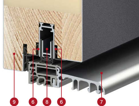
THERMO HOT 78 ajtószárny keresztmetszete takaró tömítéssel és anélkül, alumínium küszöb
