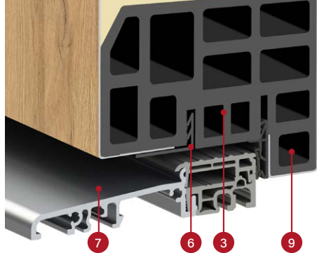
THERMO HOT 88 ajtószárny keresztmetszete takaró tömítéssel és anélkül, alumínium küszöb
