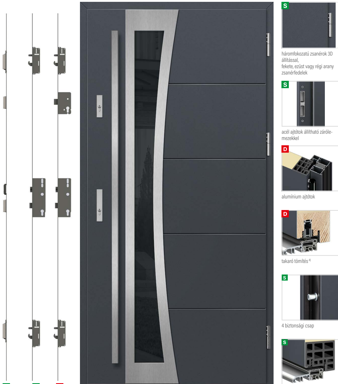
BAZYLEA 5, selyem antracit, LABEL INOX
